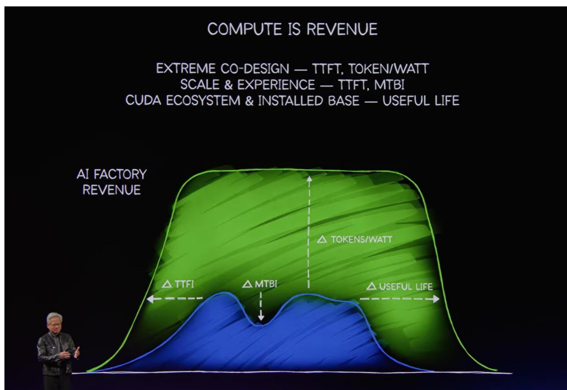
圖 4：Tokens/Watt 為關鍵
